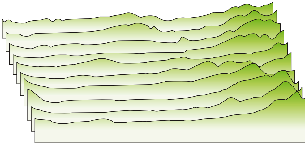
Quasi-Blockbild mittels einer Profilstaffel
