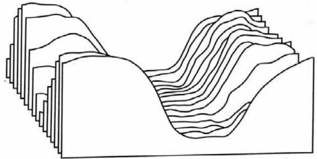
Quasi-Blockbild mittels einer Profilstaffel
